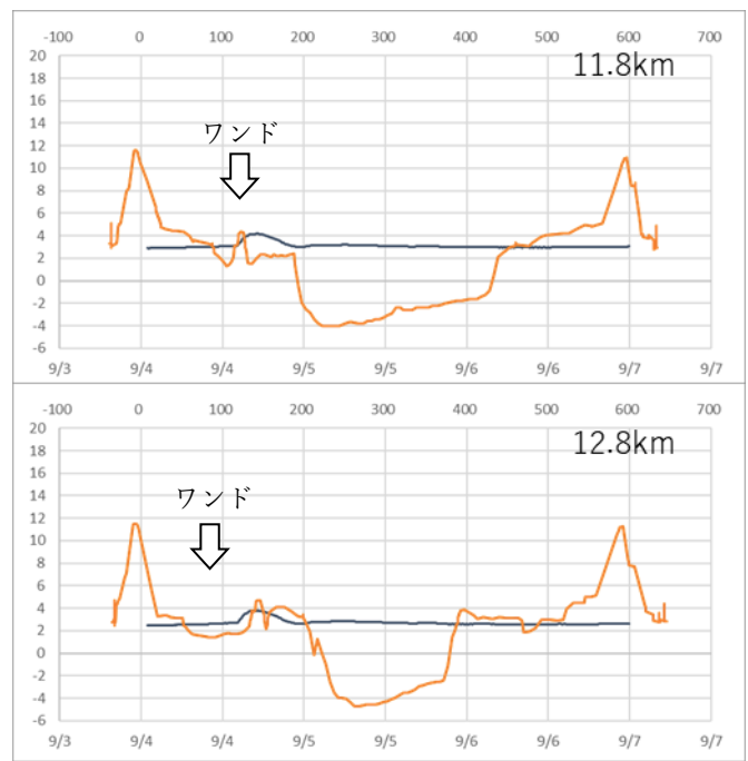
図5 平成30年9月台風21号における11.8km,12.8km地点の水位ハイドロ
